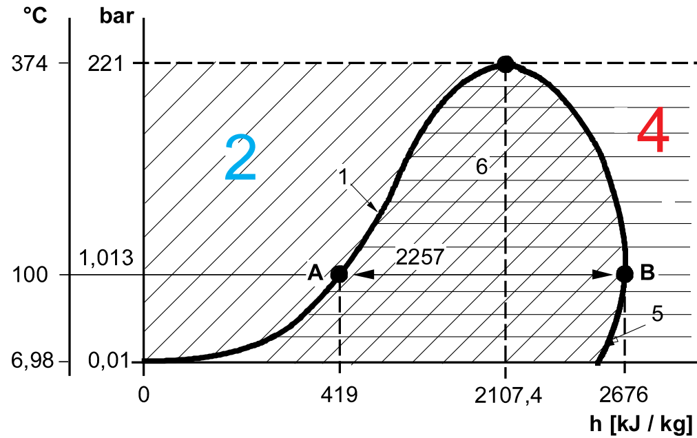
Druck-Enthalpie-Diagramm für Wasser
